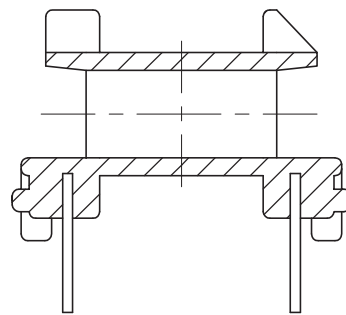
SEC. A-A
